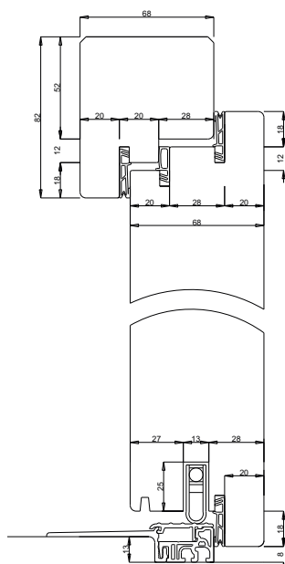
Anschlägschiene BKV Eifel RS 85 T
