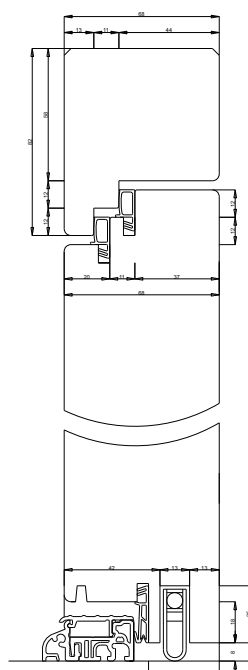
Anschlägschiene BKV Eifel 40 T
