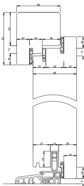
Anschlägschiene BKV Eifel 70 T
